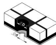
H — сквозное отверстие для крепления болтами
